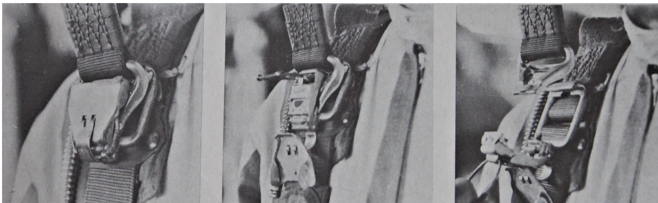
1½-shot olkalukko suljettuna, suojakansi avattuna ja vaijerilenkistä vedon jälkeen irrotettuna. Kuva: via Ilmailu
