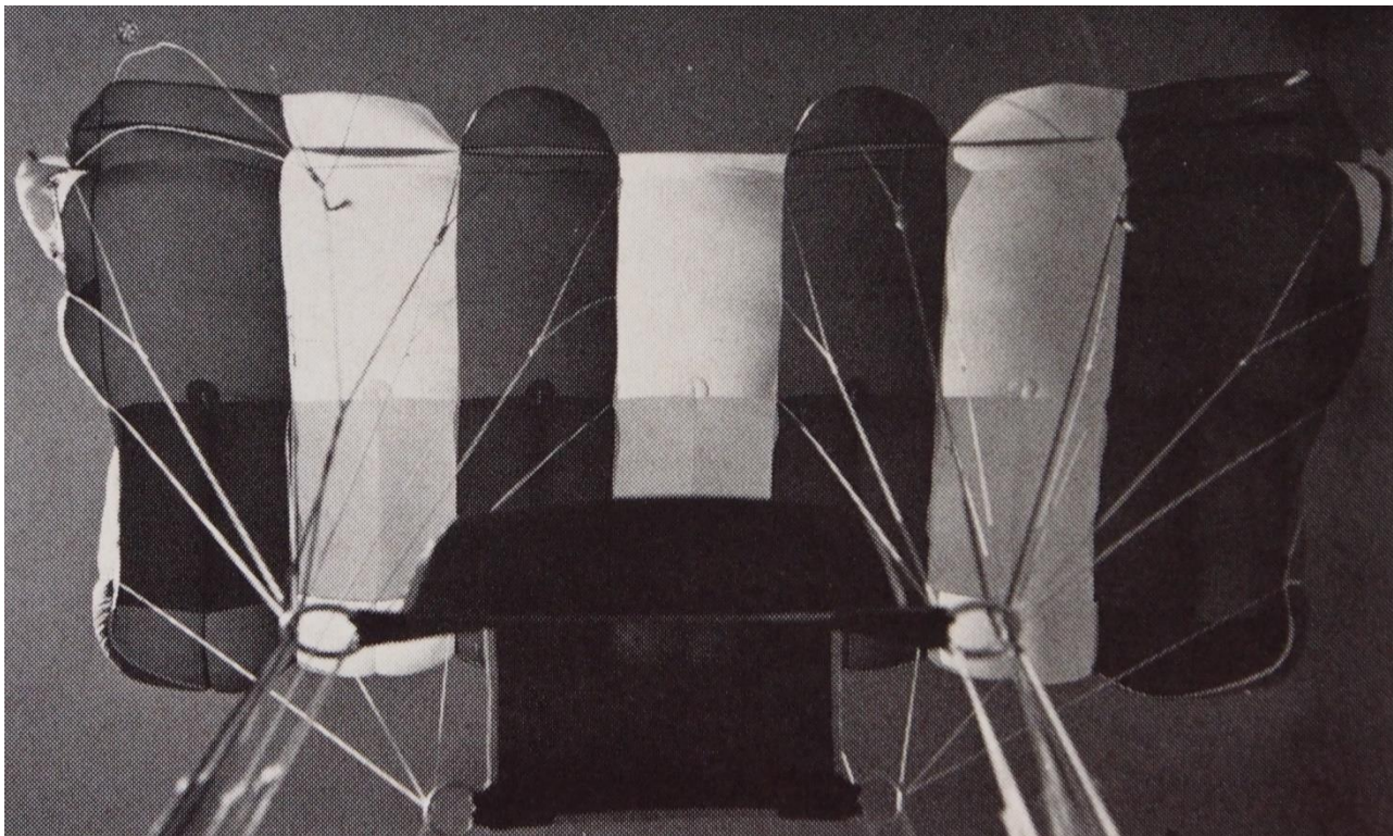
Patjavarjon liukuhidastin eli slider, kuvassa vielä noin punosten puolivälissä. Kupu on jo täysin kehittynyt ja slider jatkaa valumistaan kantohihnojen kantorenkaisiin saakka. Kuva: Spotter Magazine via Laskuvarjourheilu
